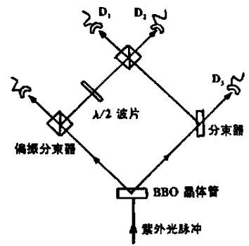
图 7 演示空间分离 3 光子 GHZ 纠缠态的实验装置
