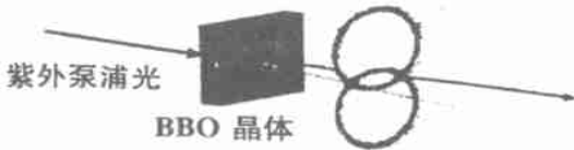
图 4 类参量下转换产生的由偏振纠缠光子组成的定向光束
