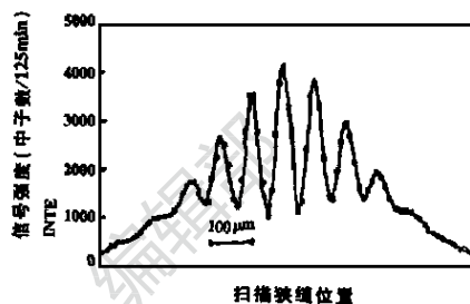
图 1 中子双狭缝实验结果
